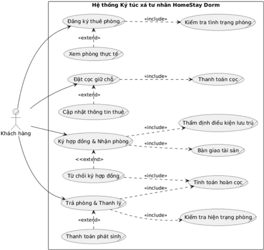
Hình 1: Mô hình Use Case nghiệp vụ
