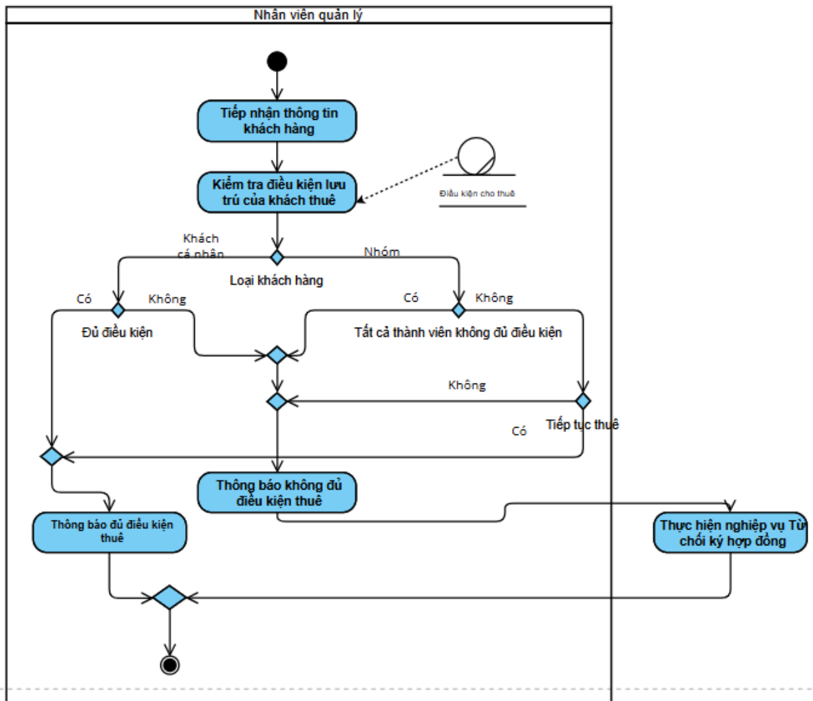
Hình 9: Activity Diagram cho Thẩm định điều kiện lưu trú
