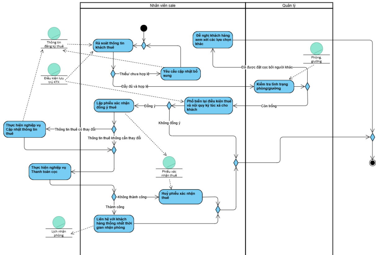
Hình 5: Activity Diagram cho Đặt cọc giữ chỗ
