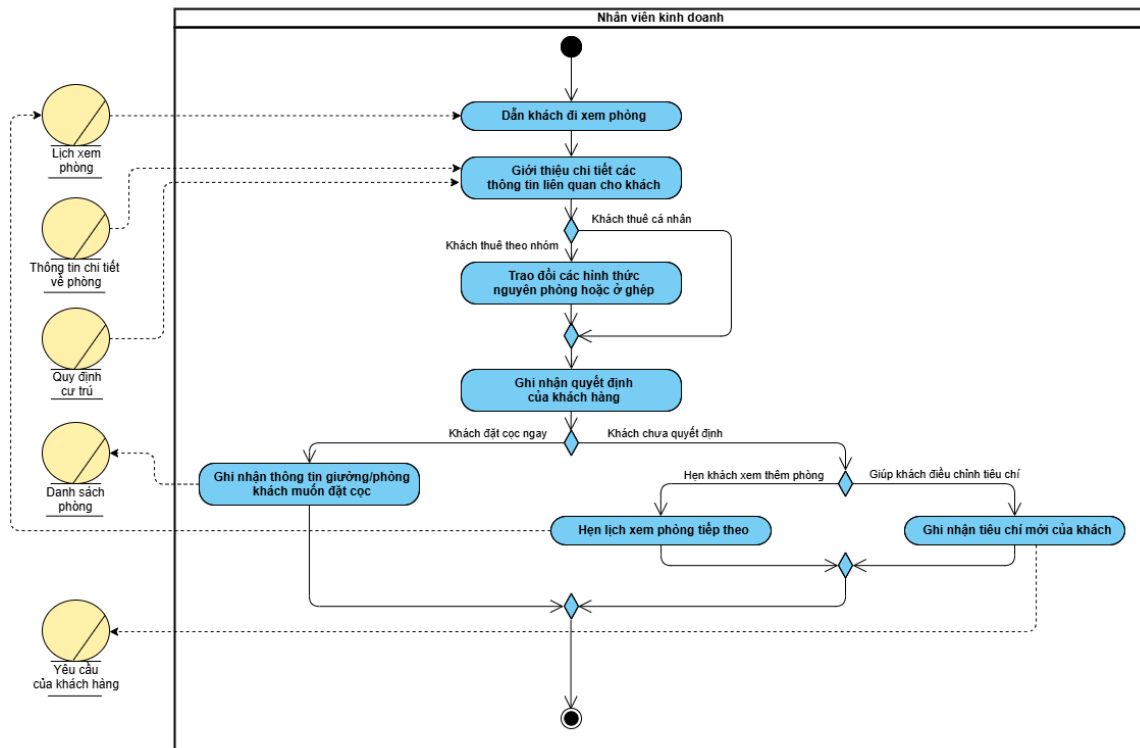
Hình 4: Activity Diagram cho Xem phòng thực tế
