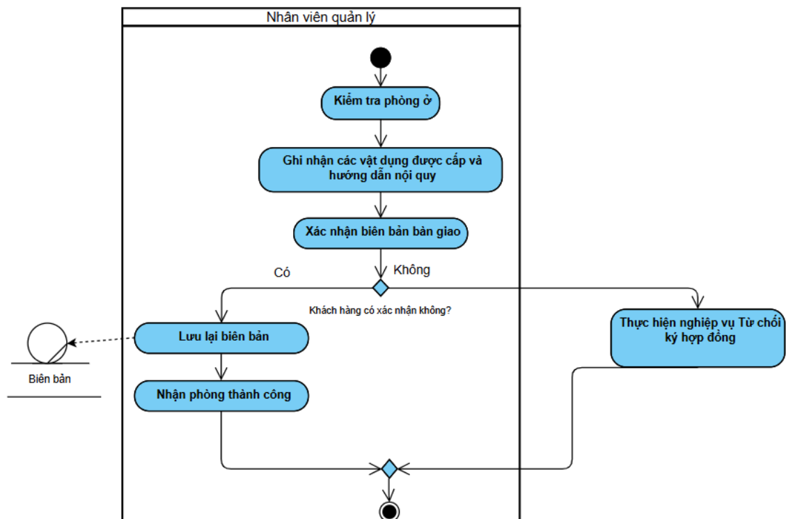
Hình 11: Activity Diagram cho Bàn giao tài sản
