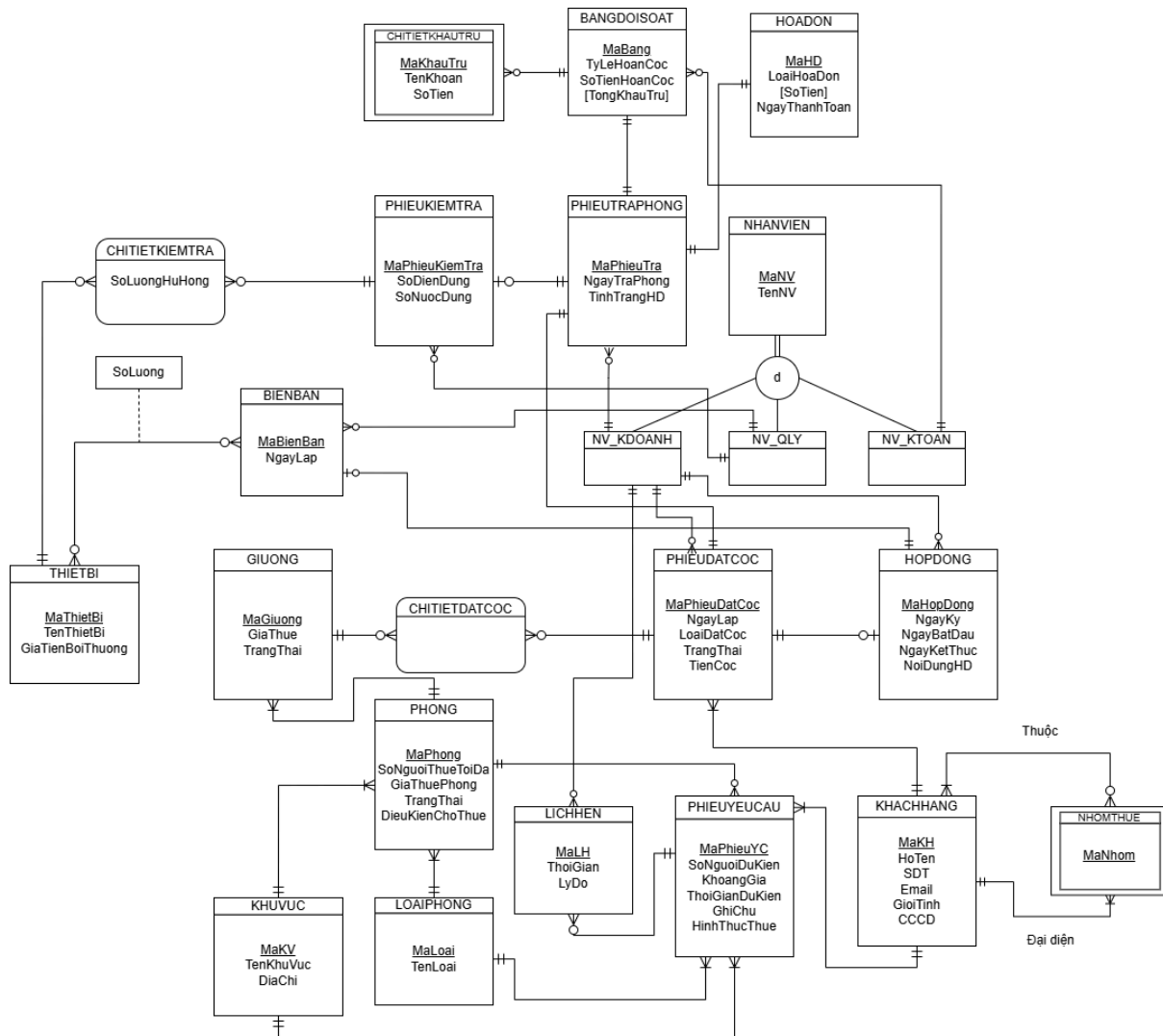
Hình 16: ERD của hệ thống
