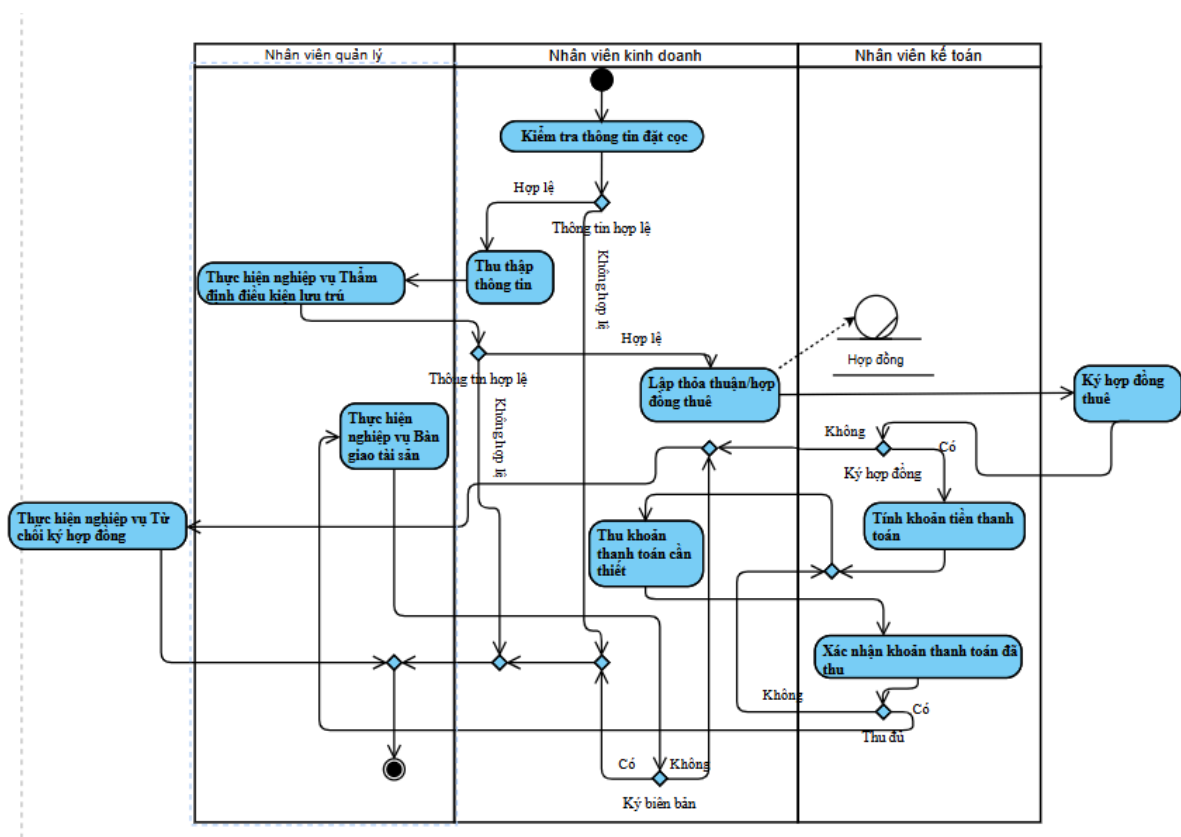
Hình 8: Activity Diagram cho Ký hợp đồng & Nhận phòng
