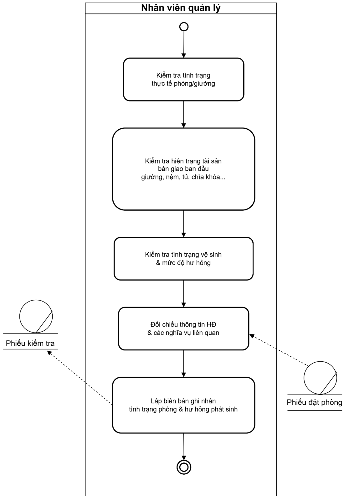
Hình 13: Activity Diagram cho Kiểm tra hiện trạng phòng
