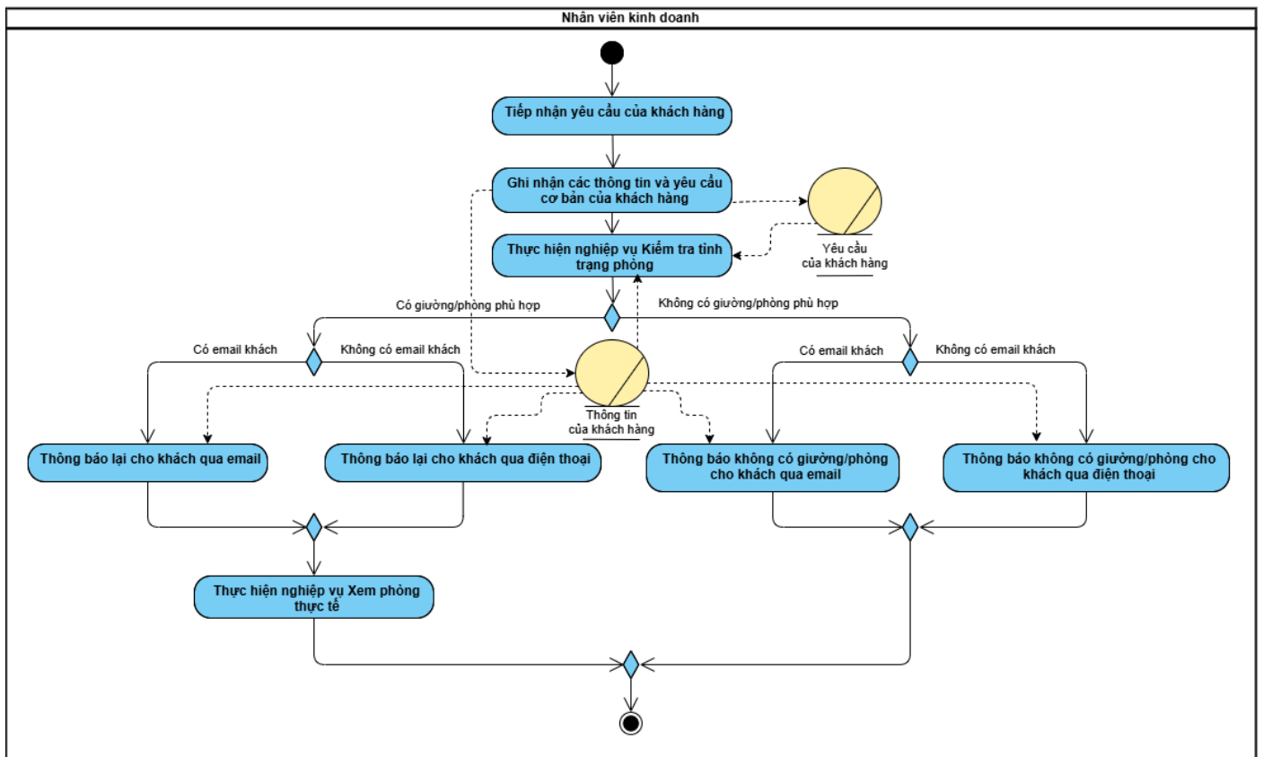
Hình 2: Activity Diagram cho Đăng ký thuê phòng
