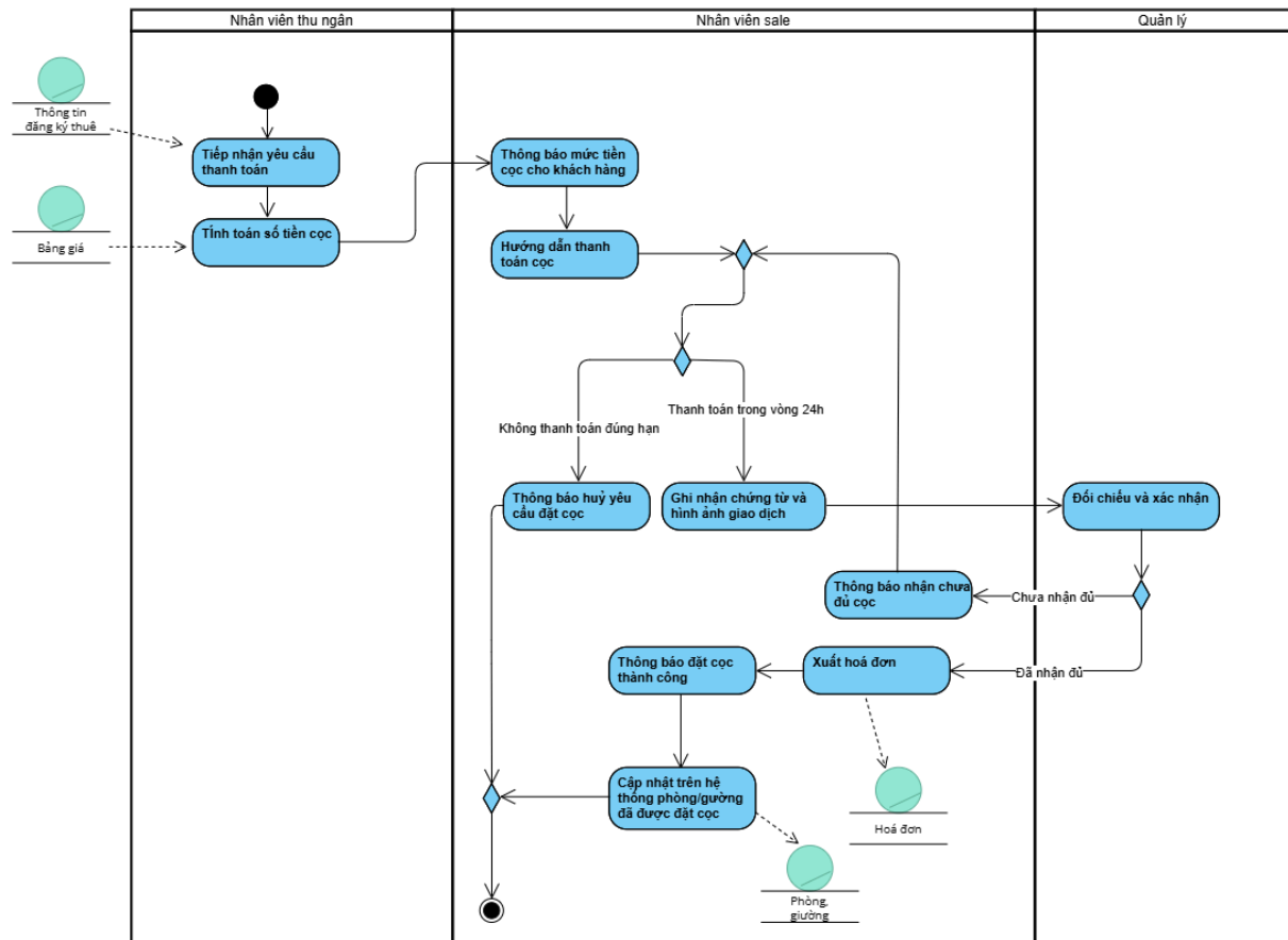
Hình 6: Activity Diagram cho Thanh toán cọc
