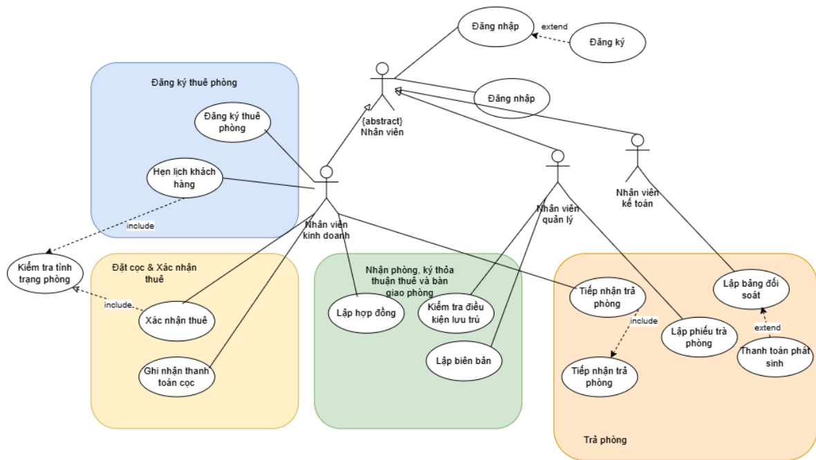
Hình 17: Use Case hệ thống
