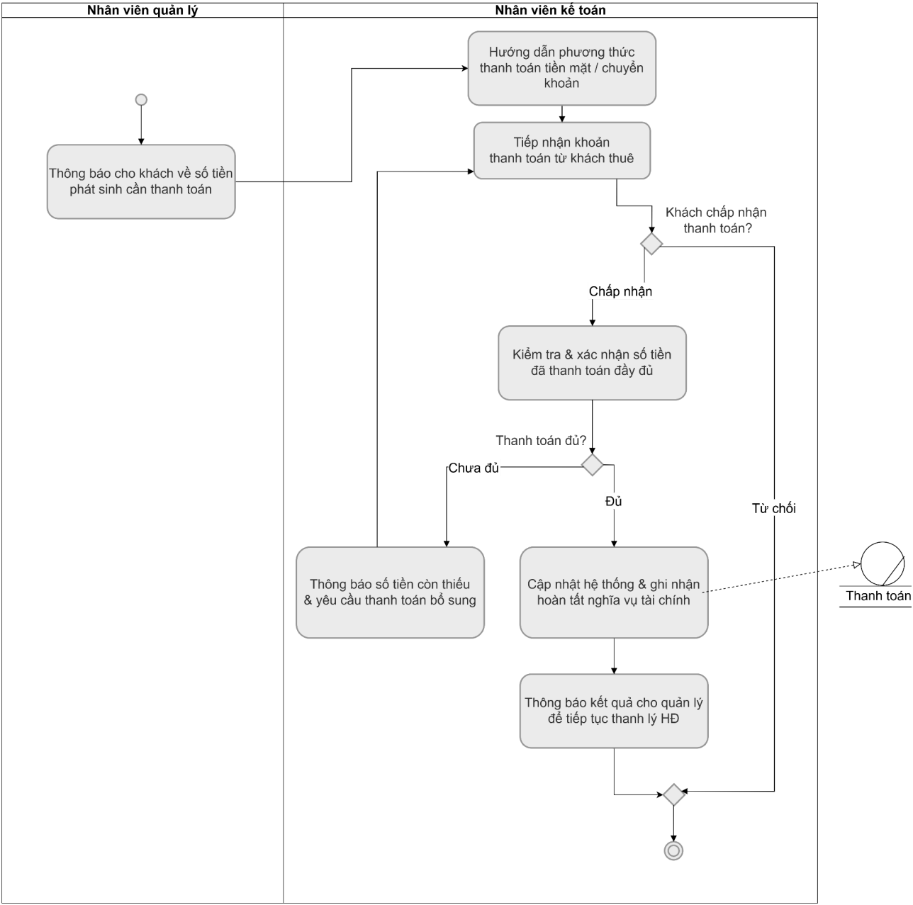
Hình 15: Activity Diagram cho Thanh toán phát sinh
