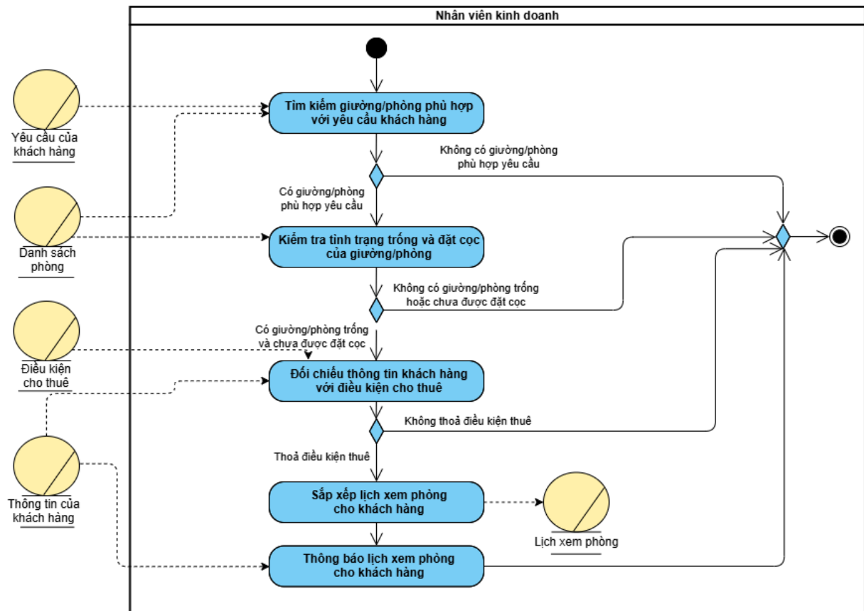
Hình 3: Activity Diagram cho Kiểm tra tình trạng phòng
